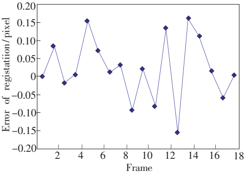
图 5 配准误差曲线
