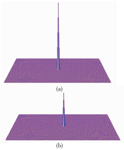
图 1 相位相关函数. (a) (x_0,y_0)=(0,0) , (b) (x_0,y_0)=(0.5,0)
