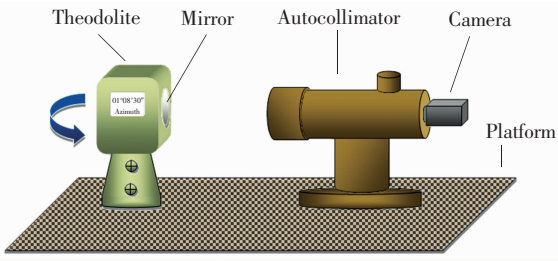
图 3 光斑图像配准实验装置 Fig. 3 Setup of experimental system
